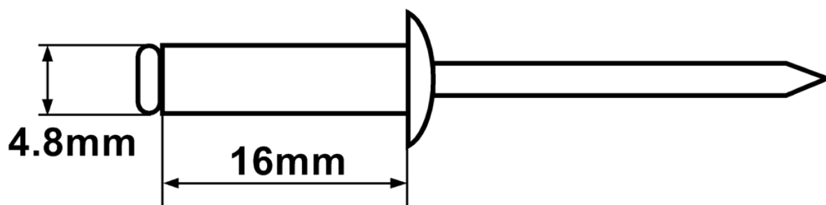
Рисунок 1-чертеж заклепки
